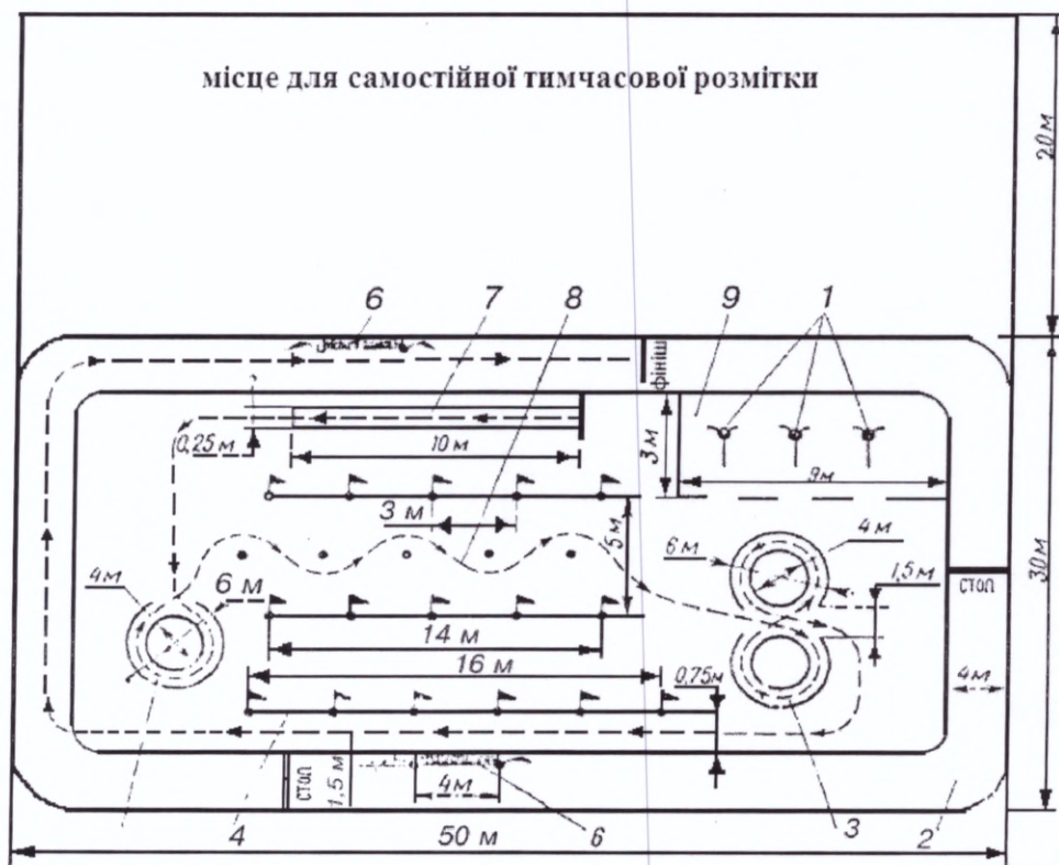
Малюнок 1 – Схема майданчика із розміткою
