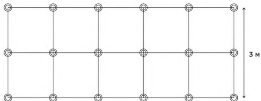
Елемент поля гвинтових паль
